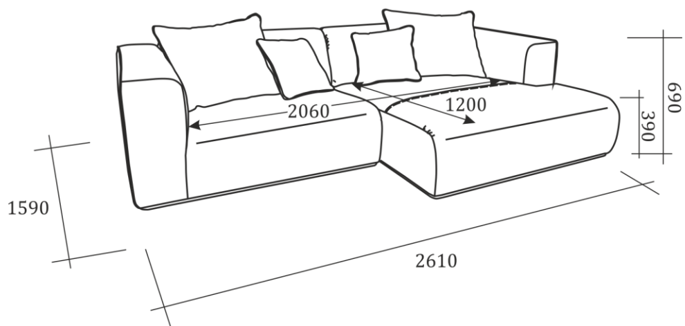
A5П Диван угловой правый
